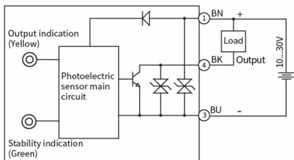
NPN
