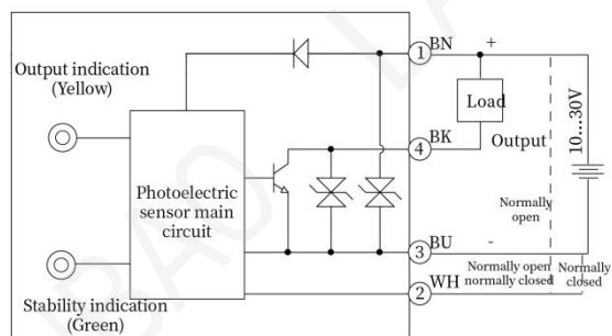
NPN
